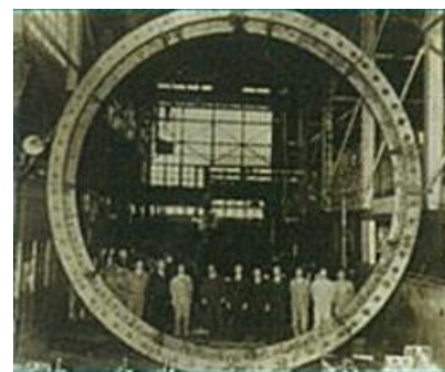
4. 関門トンネル鑄鉄セグメント(1939年)
